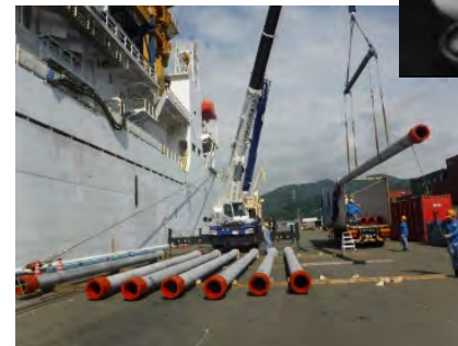
6,000m揚泥管組立・搭載関連 (出典) 内閣府
